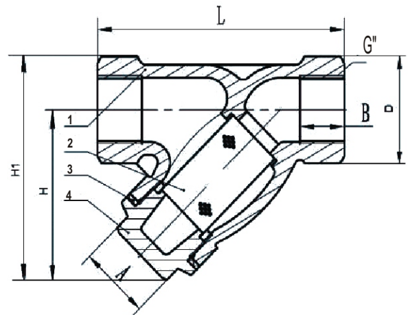
Чертеж габаритный фильтра ABRA-ФММ (размеры в таблице):
